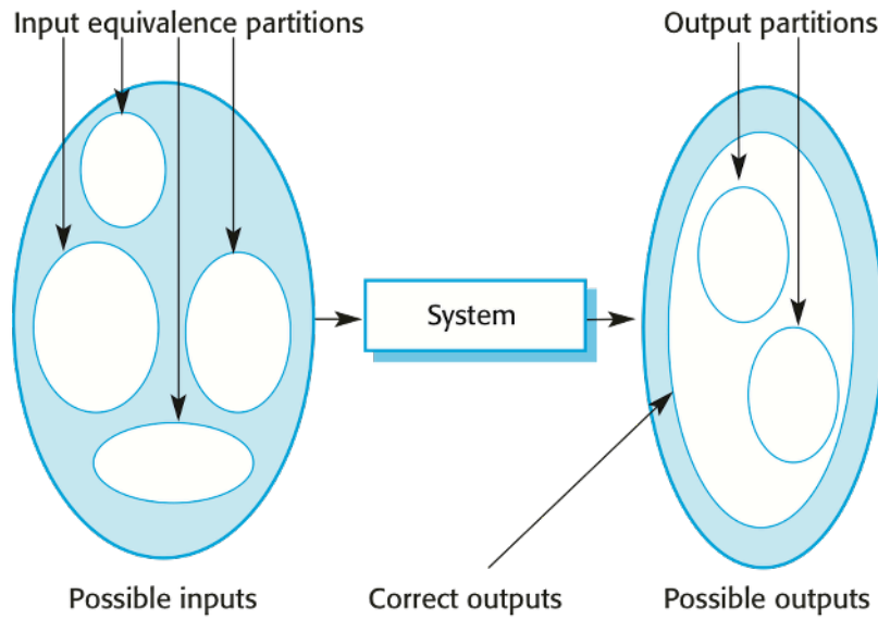
Einteilung in Äquivalenzklassen (Quelle: I. Sommerville: Software Engineering)
