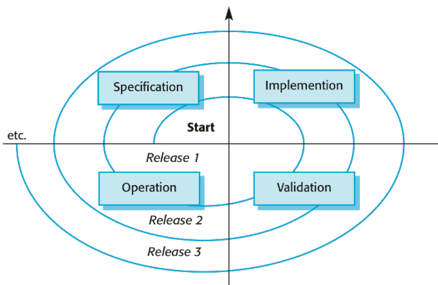
Spiralmodell (Quelle: I. Sommerville: Software Engineering)
